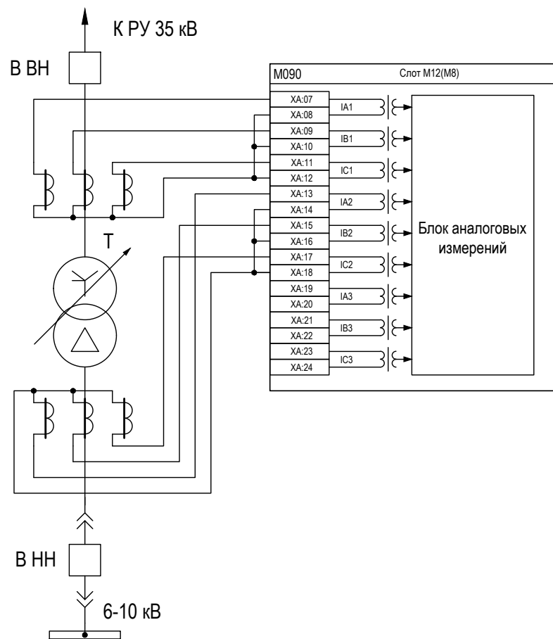
Рисунок Г.1 – Подключение аналоговых цепей трансформаторов тока двухобмоточного трансформатора 35 кВ к устройству
