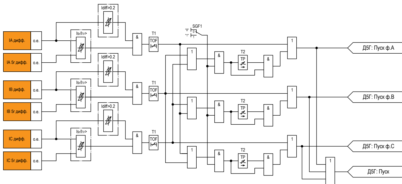
Рисунок 2.6 – Функциональная схема логики Д5Г
