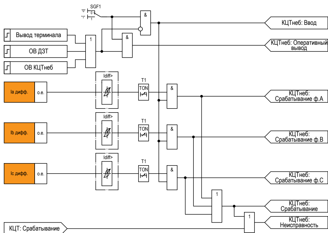
Рисунок 2.9 – Функциональная схема логики КЦТнеб
