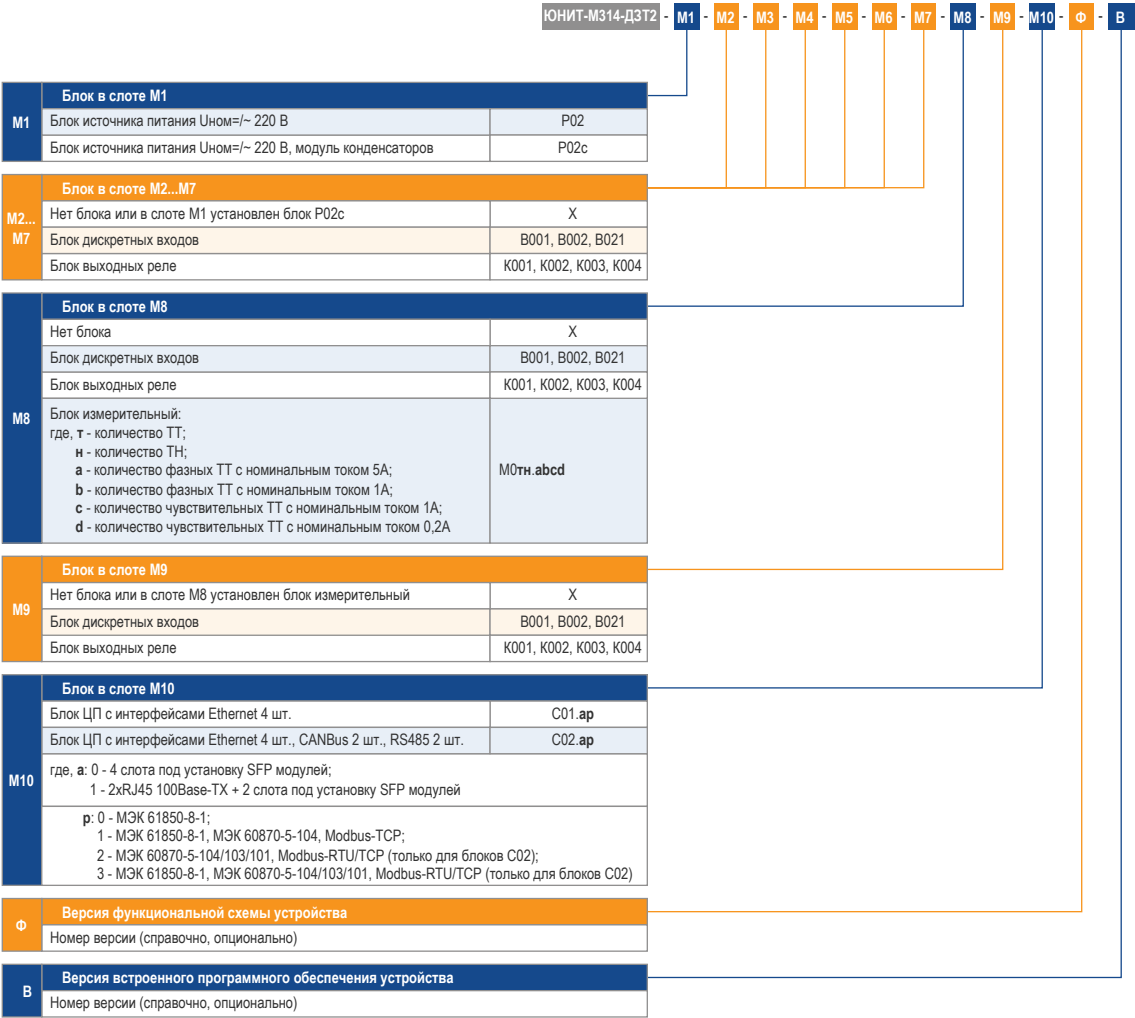
Рисунок Б.1 – Код заказа устройства «ЮНИТ-М314-Д3Т2»
